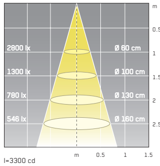
halogen reflector, PAR 30 - E27, 100W, 30°
