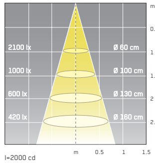
halogen reflector, PAR 30 - E27, 75W, 30°
